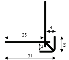
134226 Buitenhoekprofiel 4/4100 anod (+T) External corner 4/4100 anod (+T) Außeneckprofil 4/4100 elox (+T)
